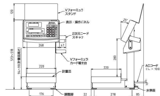
外観寸法
